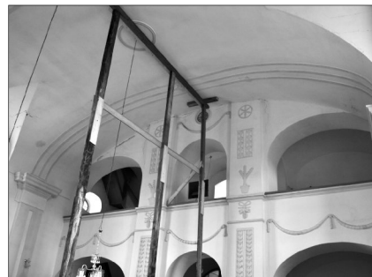
A KISPEREGI TEMPLOM ALÁTÁMASZTOTT TETŐSZERKEZETE
